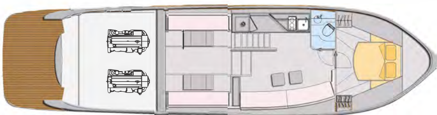
下甲板方案1
